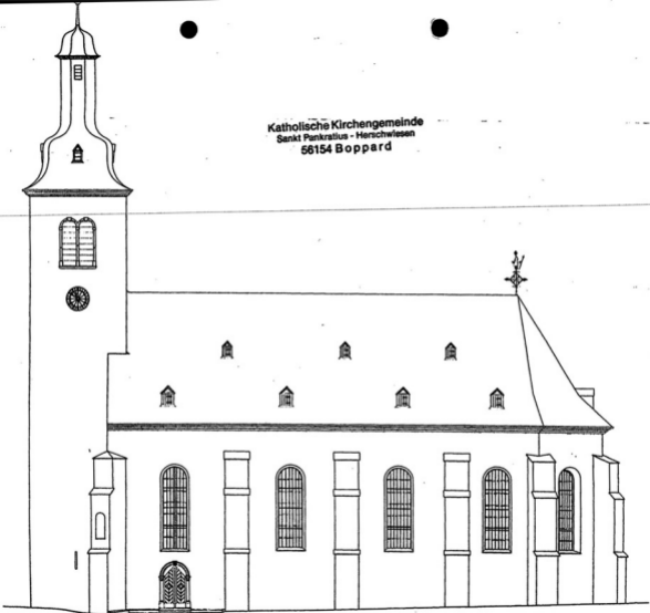
VII,4. Ortsteil Henschwiesen. Ehem. Kath. Pfarrkirche St. Pankratius. Ansicht der Südseite. Bauaufnahme im Maßstab 1:30, verkleinert auf 2/100 von Gehlhausen und Fritzsche 1928.
