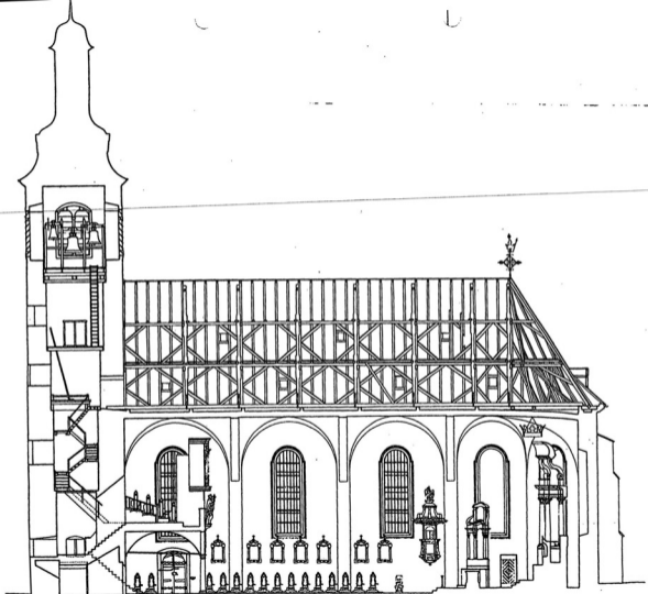
VII.3. Ortsteil Hensbrünnen. Ebern. Kath. Pfarrkirche St. Pankratius. Längsschnitt nach Norden. Bauaufnahme im Maßstab 1:150, verkleinert auf 1:1150, von Schellenkamp und Grimmelt, 1984.
